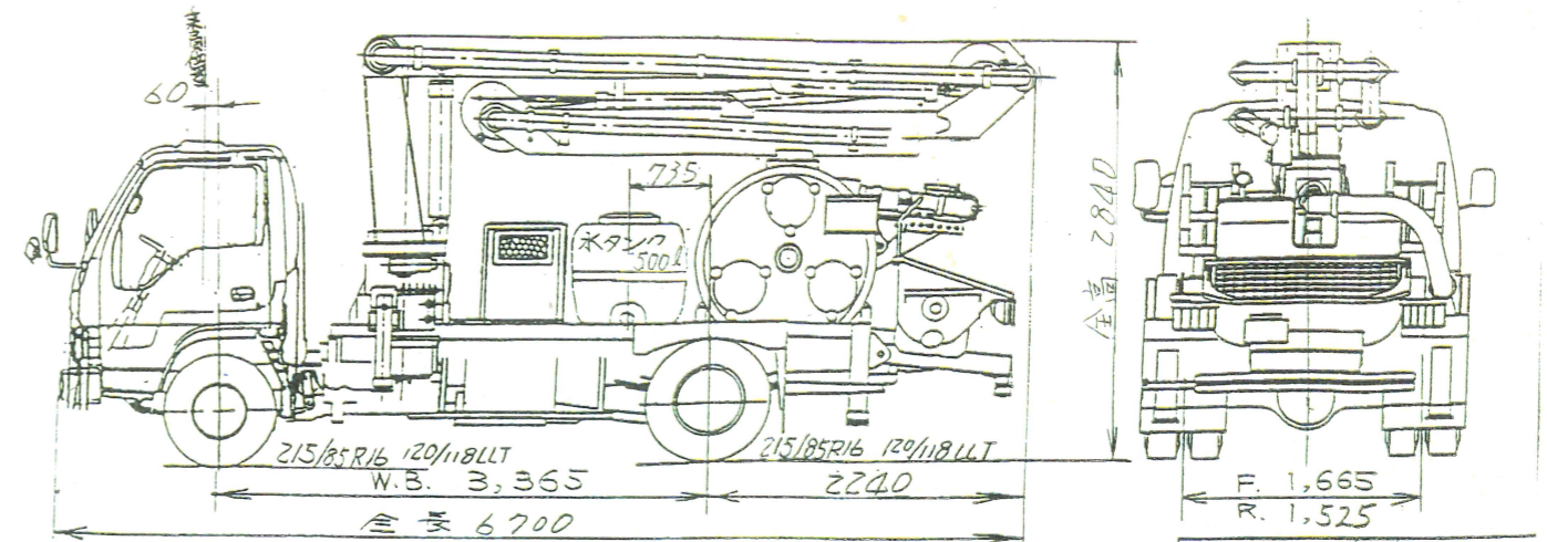
〔 外観寸法図 〕
